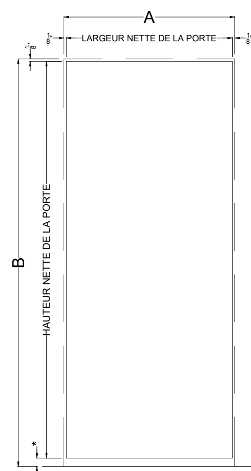
PORTE ELEVATION BF
