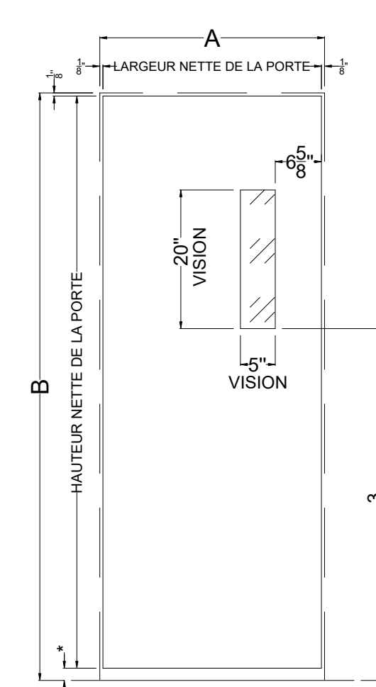
PORTE ELEVATION BNLH
