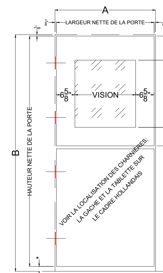
PORTE ELEVATION BH-HG (PORTE HOLLANDAISE VITRÉE)
