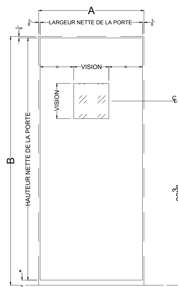
PORTE ELEVATION BV
