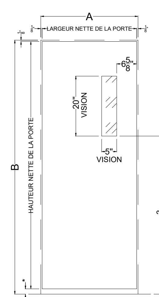
PORTE ELEVATION BNL
