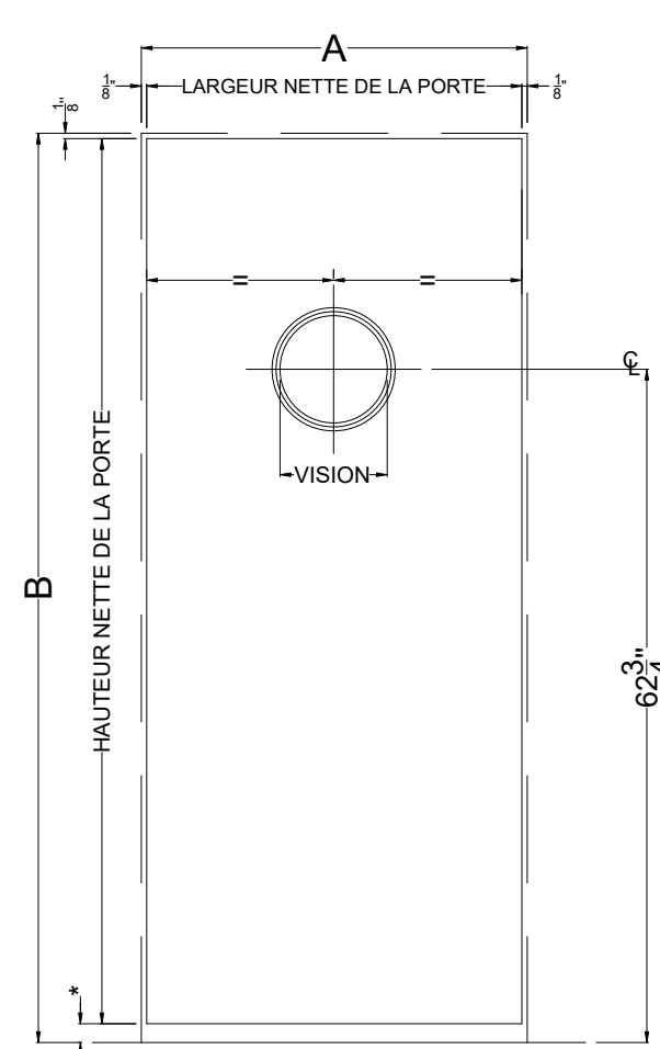
PORTE ELEVATION BR
