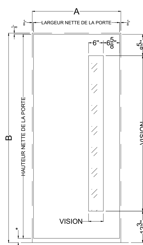
PORTE ELEVATION BNF
