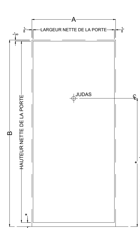
PORTE ELEVATION J1
