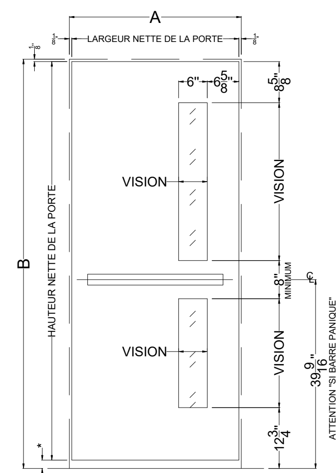
PORTE ELEVATION 2BNL
