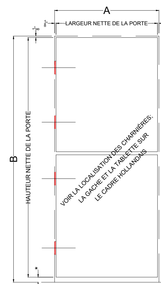
PORTE ELEVATION BH (PORTE HOLLANDAISE)
