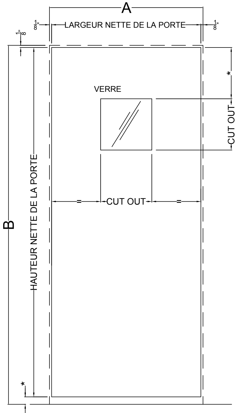
PORTE ELEVATION V
