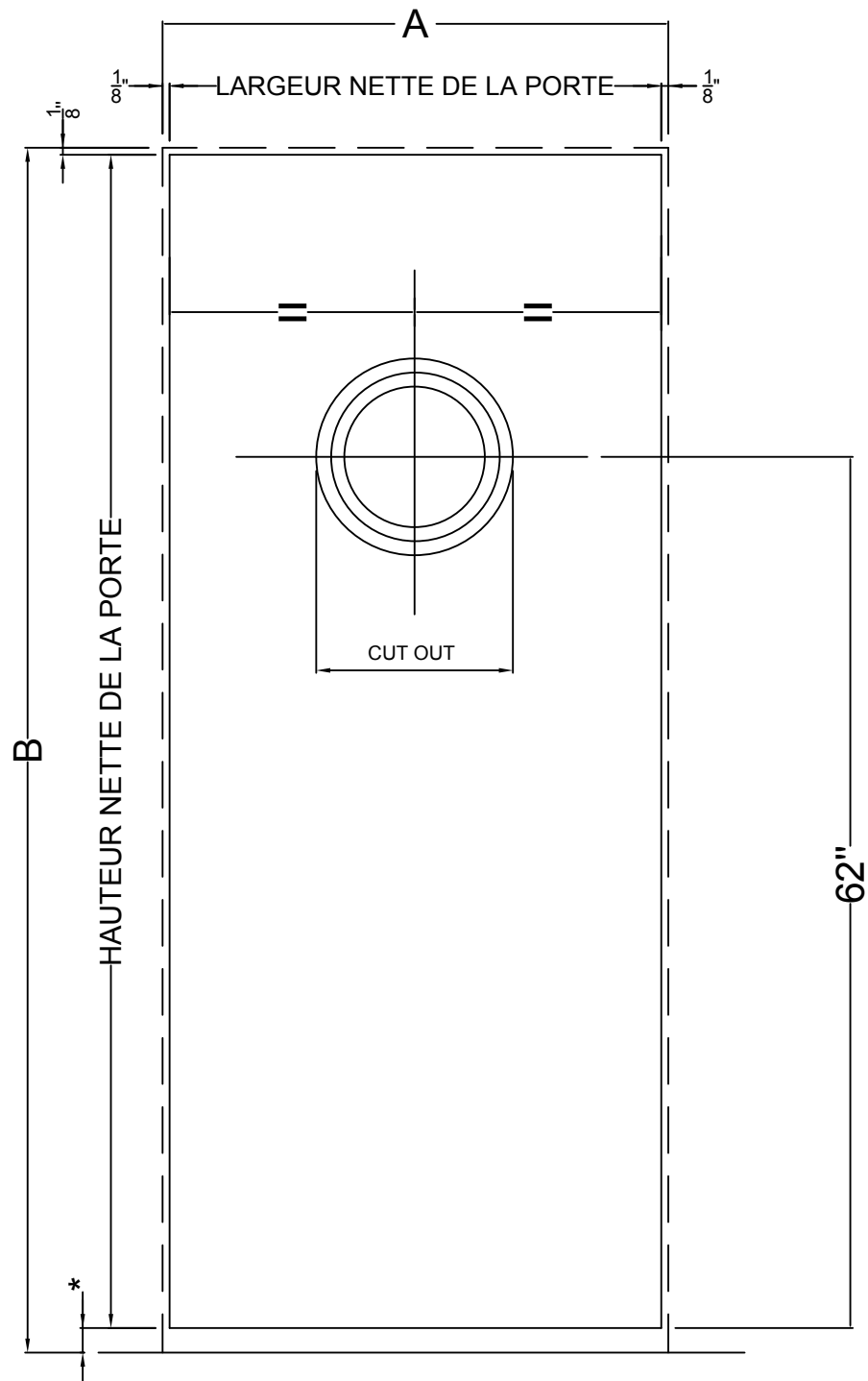
PORTE ELEVATION R
