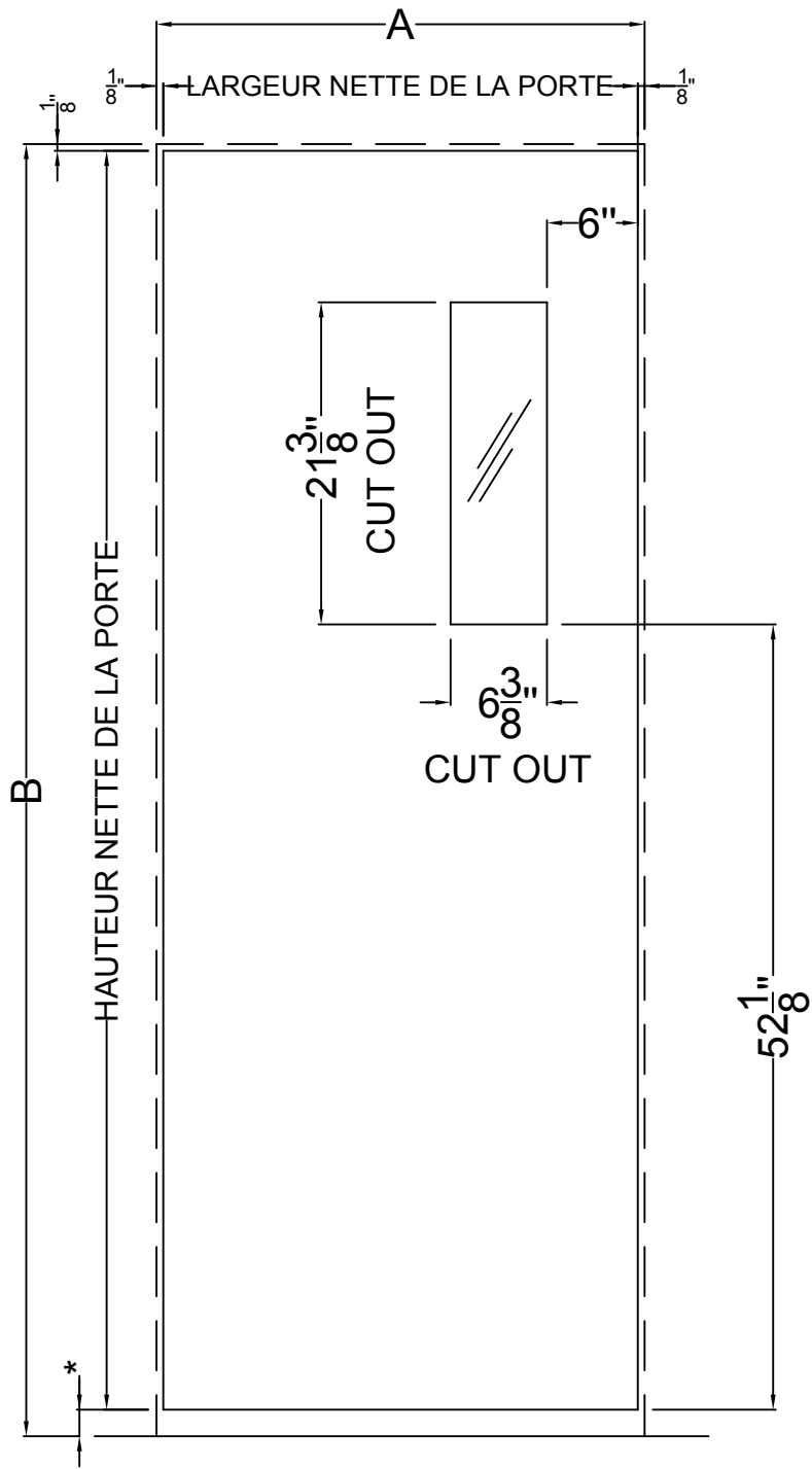
PORTE ELEVATION NL
