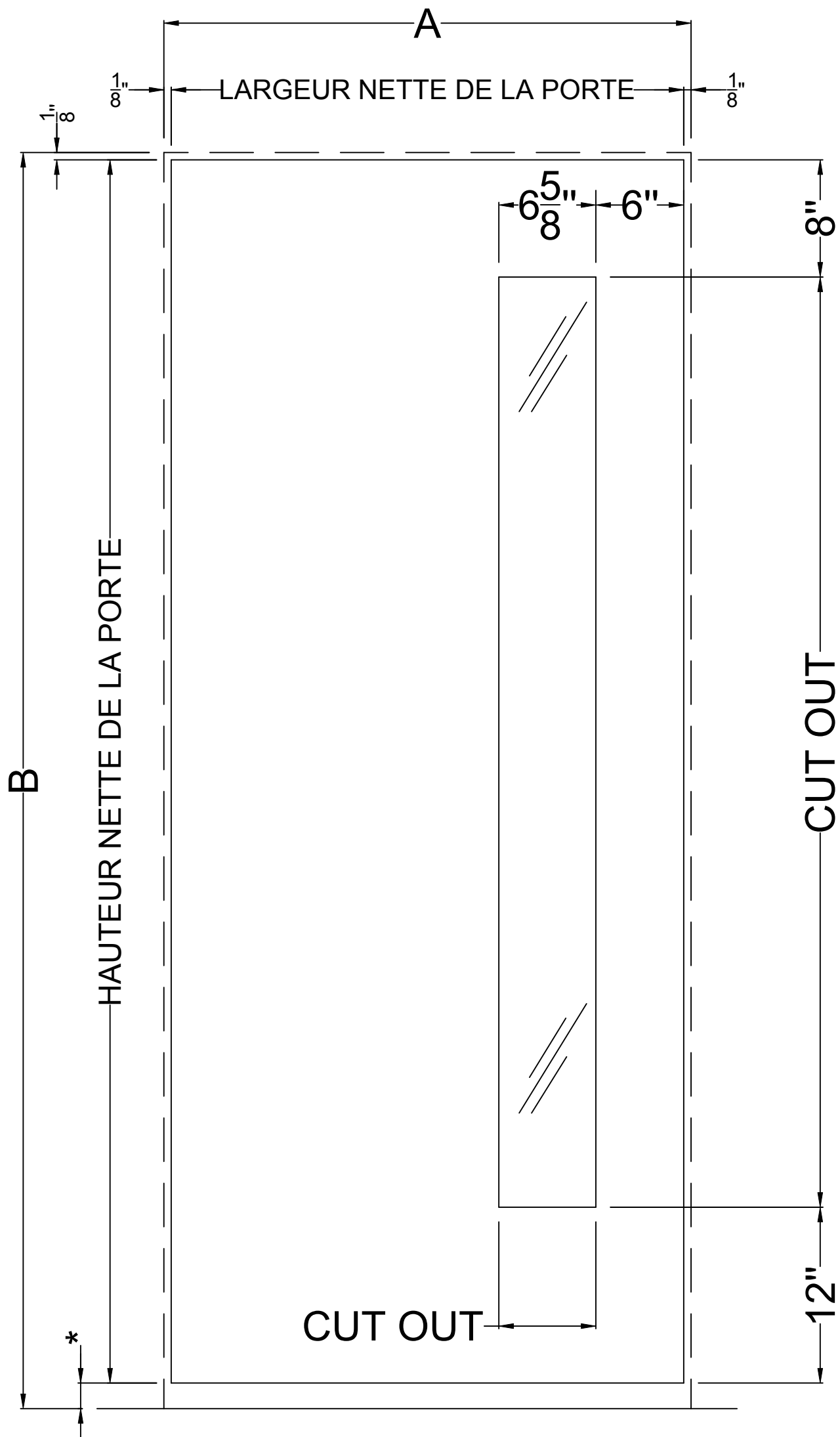
PORTE ELEVATION NF
