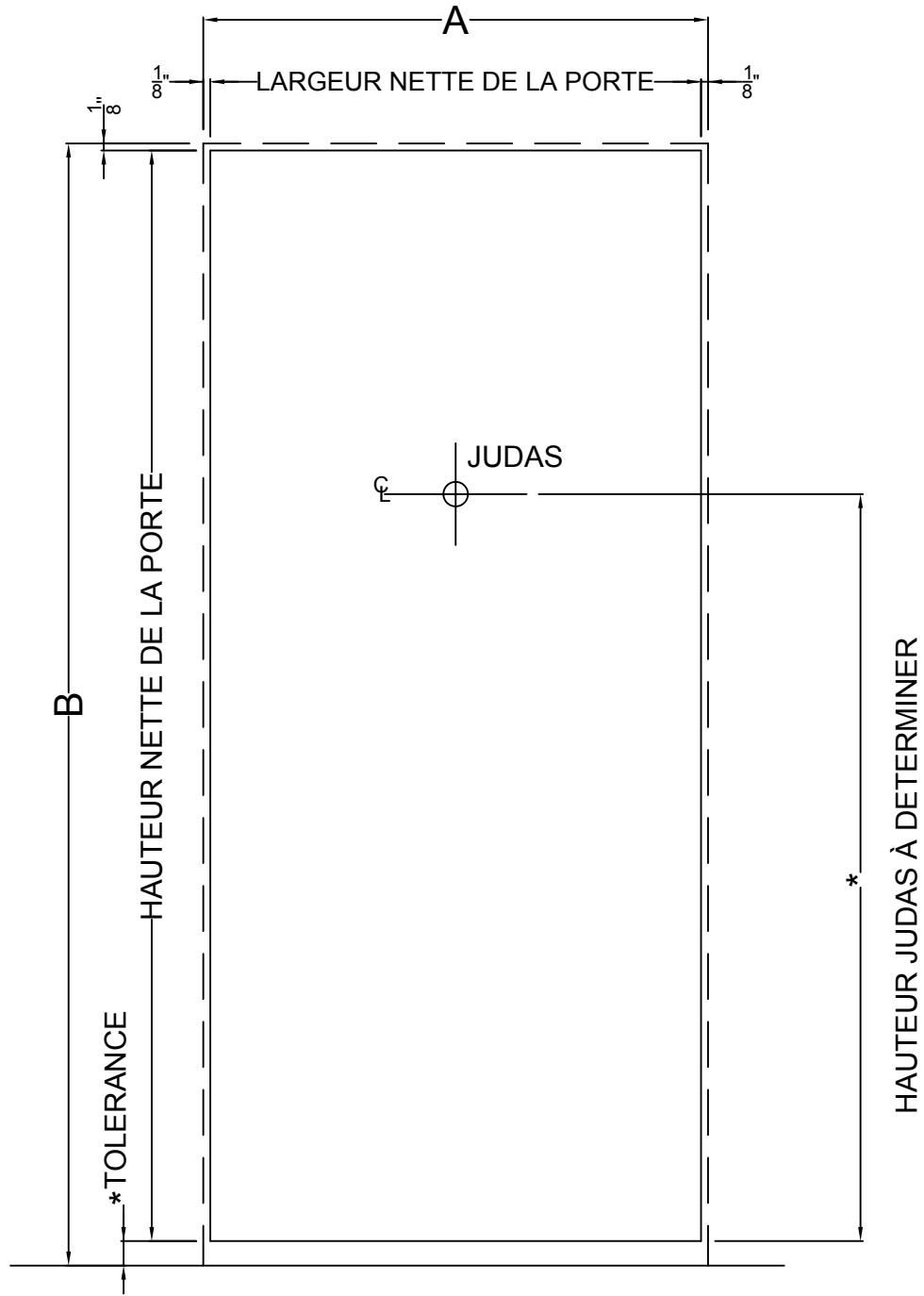
PORTE ELEVATION J1
