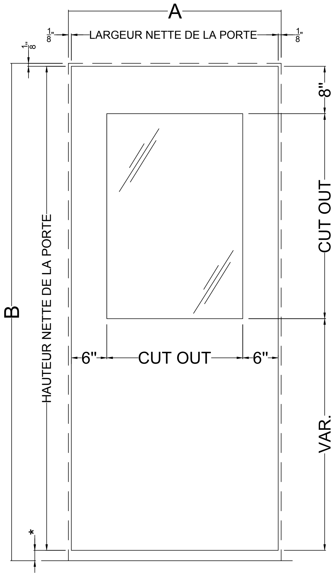
PORTE ELEVATION HG
