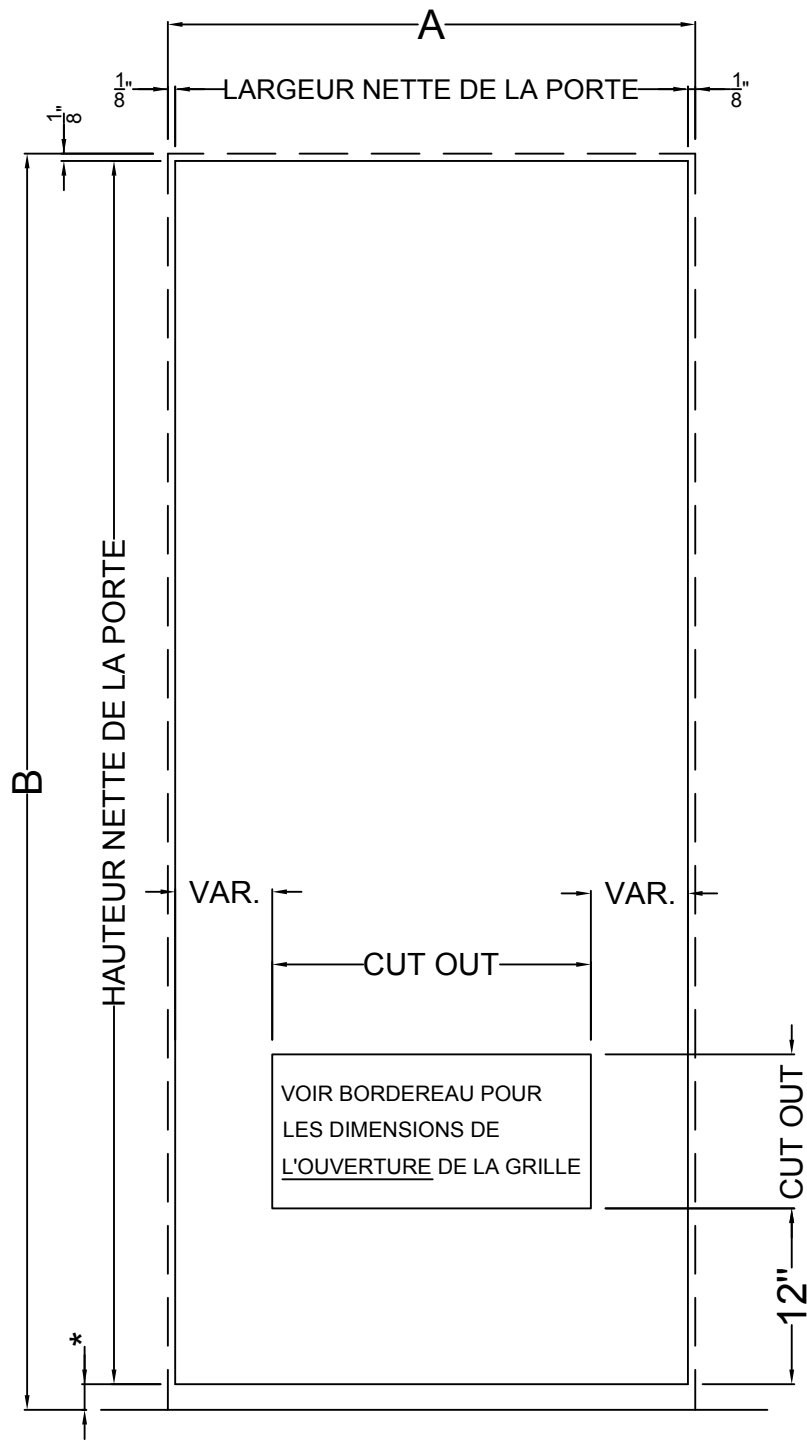
PORTE ELEVATION GR
