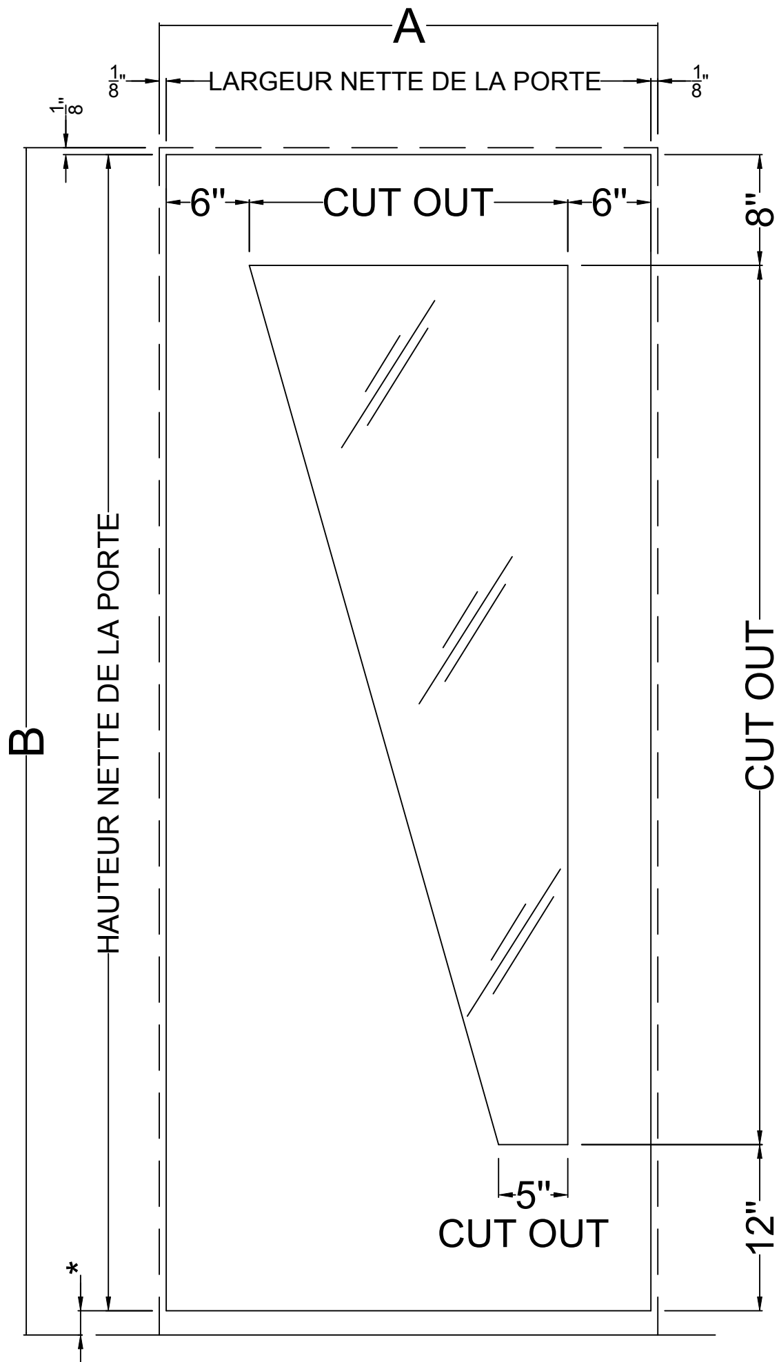
PORTE ELEVATION FS
