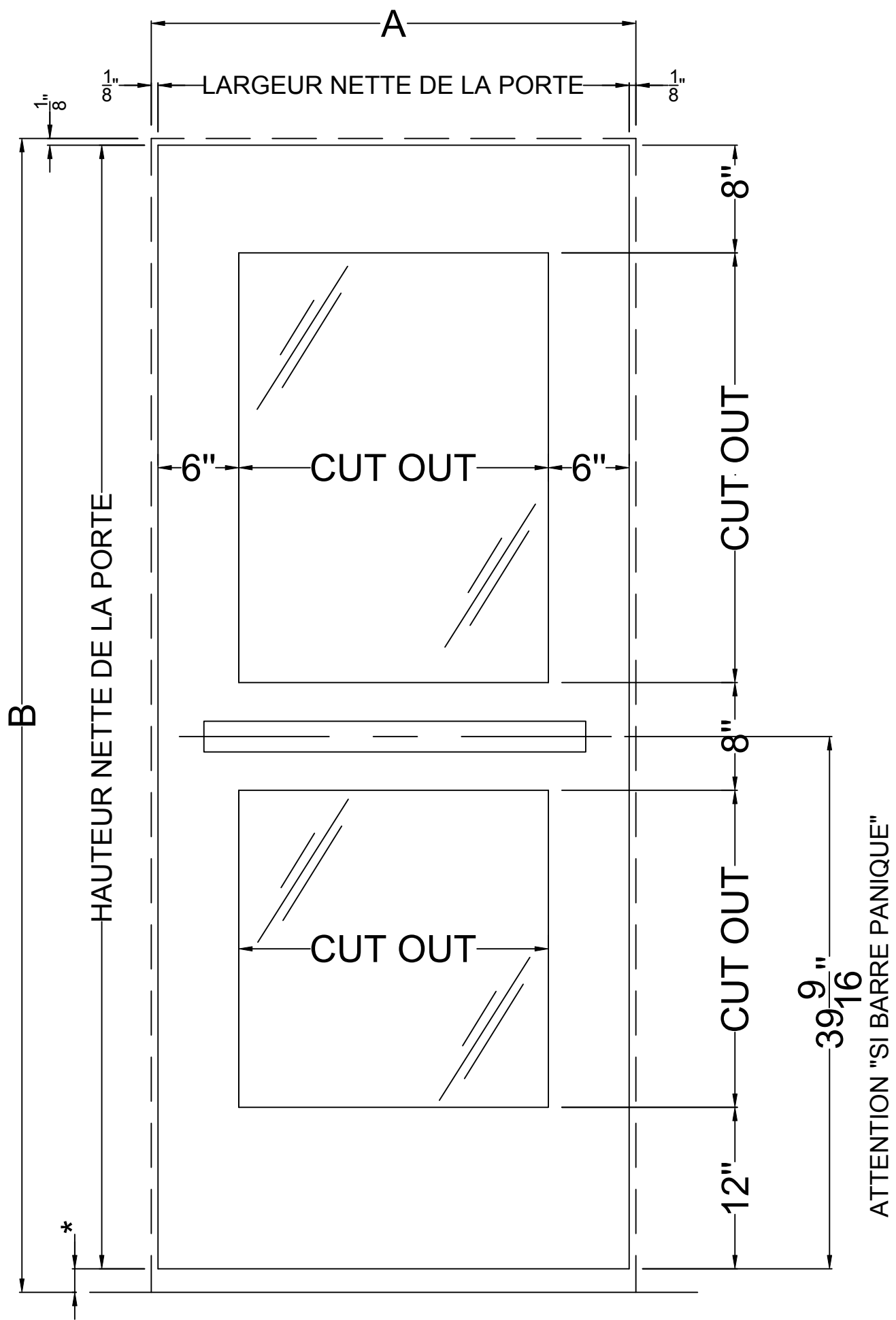
PORTE ELEVATION 2HG
