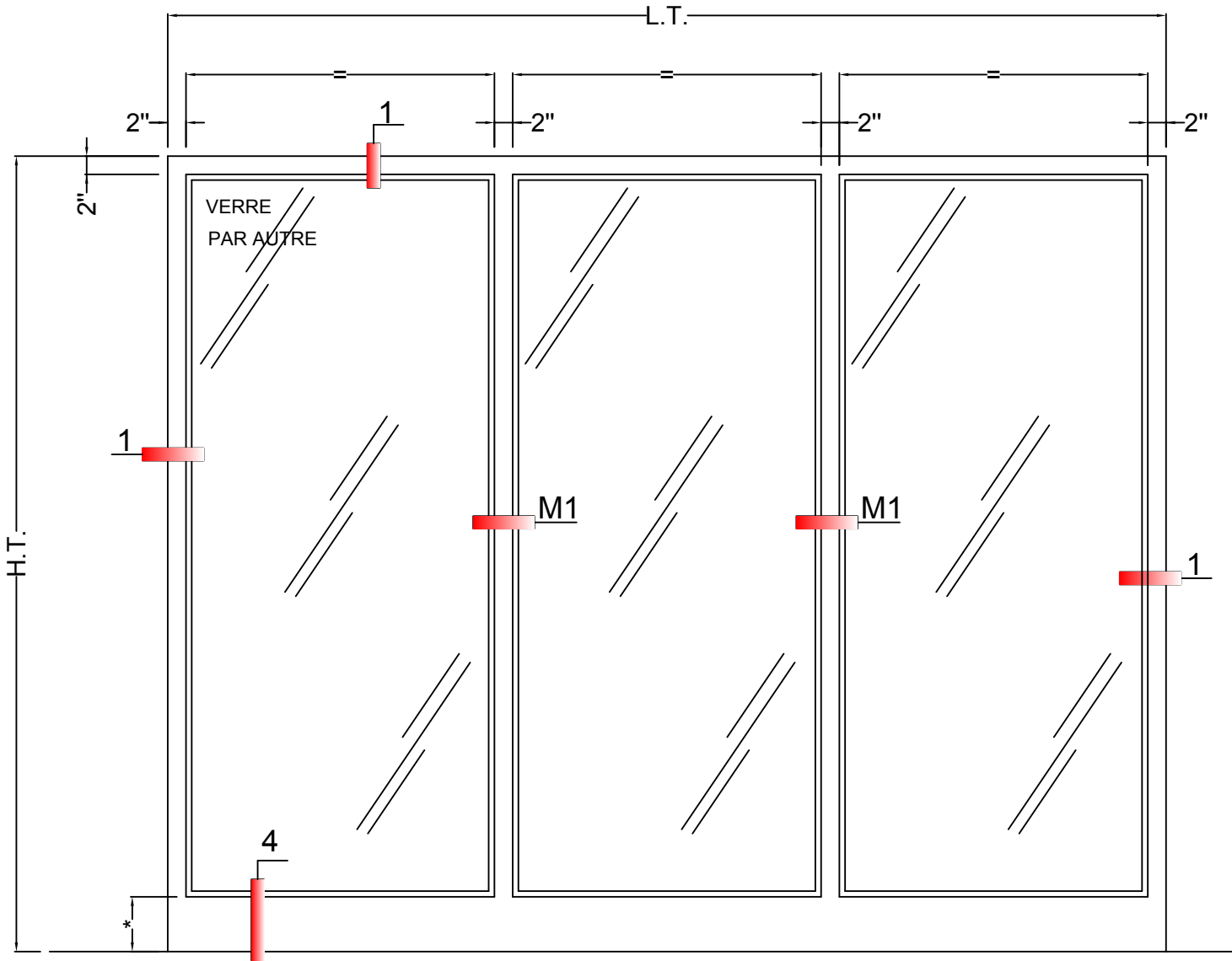
CADRE ELEVATION 6D
