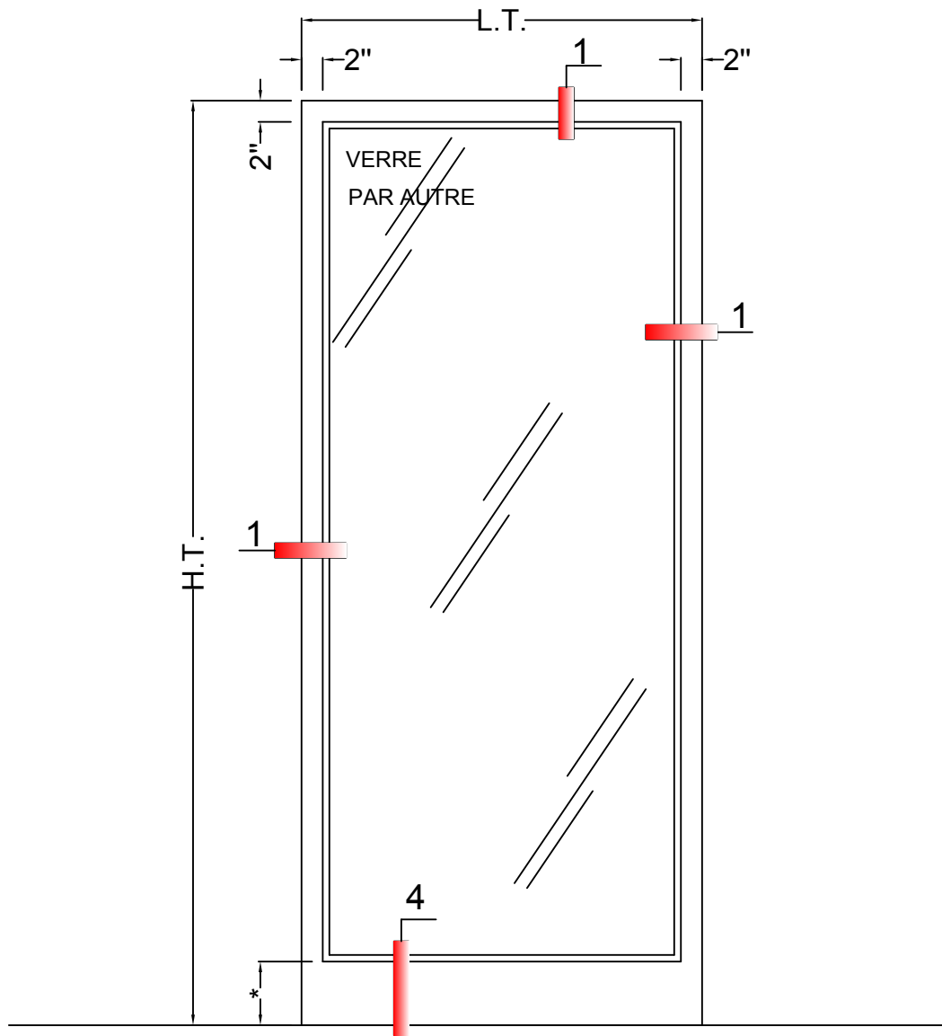
CADRE ELEVATION 6
