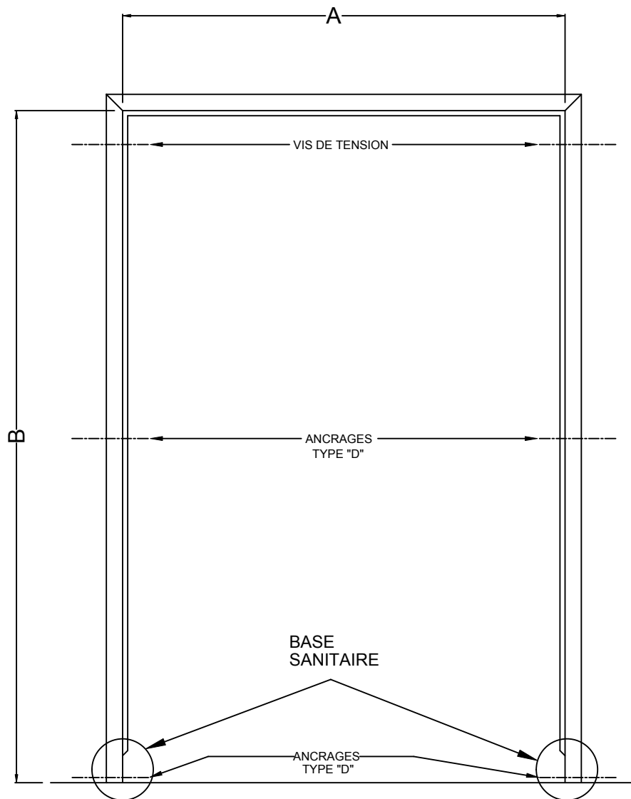
CADRE ELEVATION 2Y-BS 3 MORCEAUX-BASE SANITAIRE
