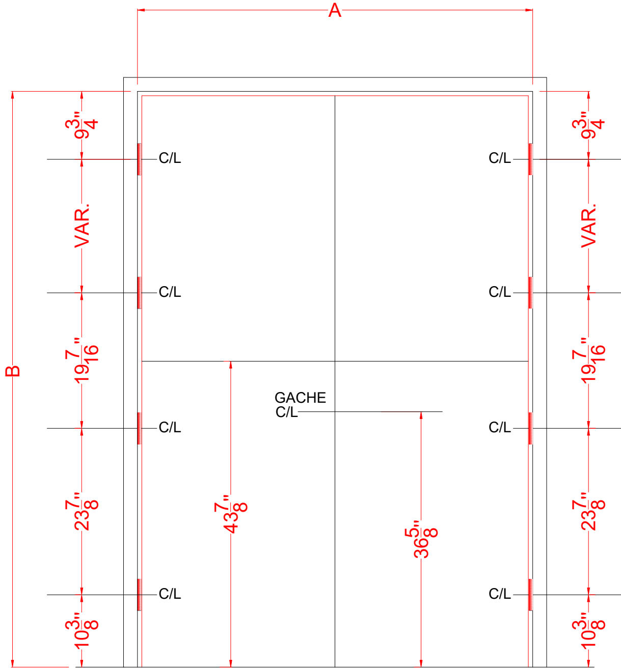
CADRE ELEVATION 2H (CADRE HOLLANDAIS)
