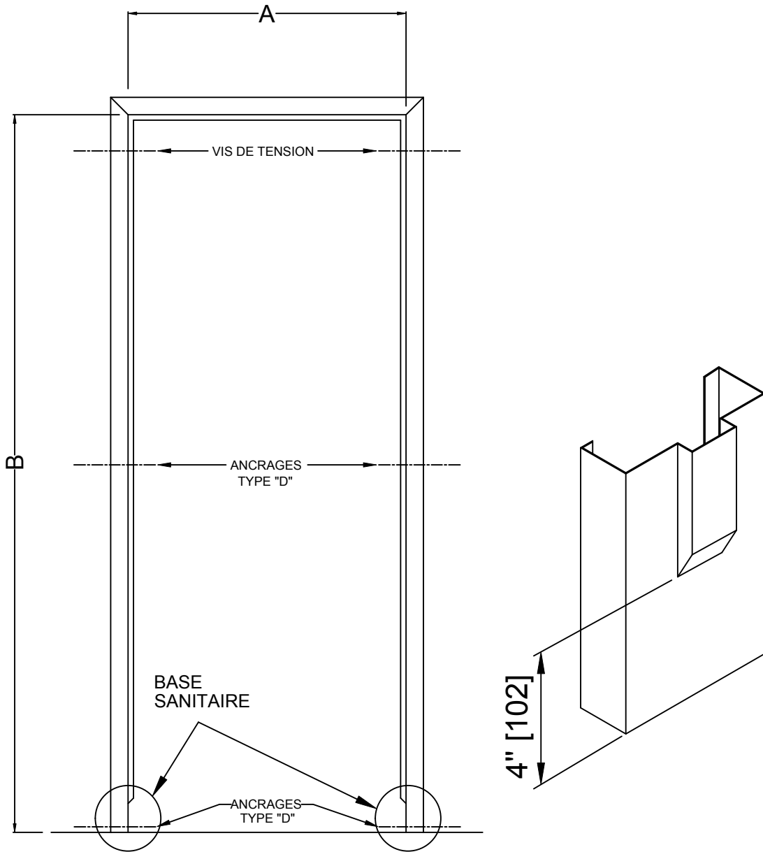
CADRE ELEVATION 1Y-BS 3 MORCEAUX-BASE SANITAIRE
