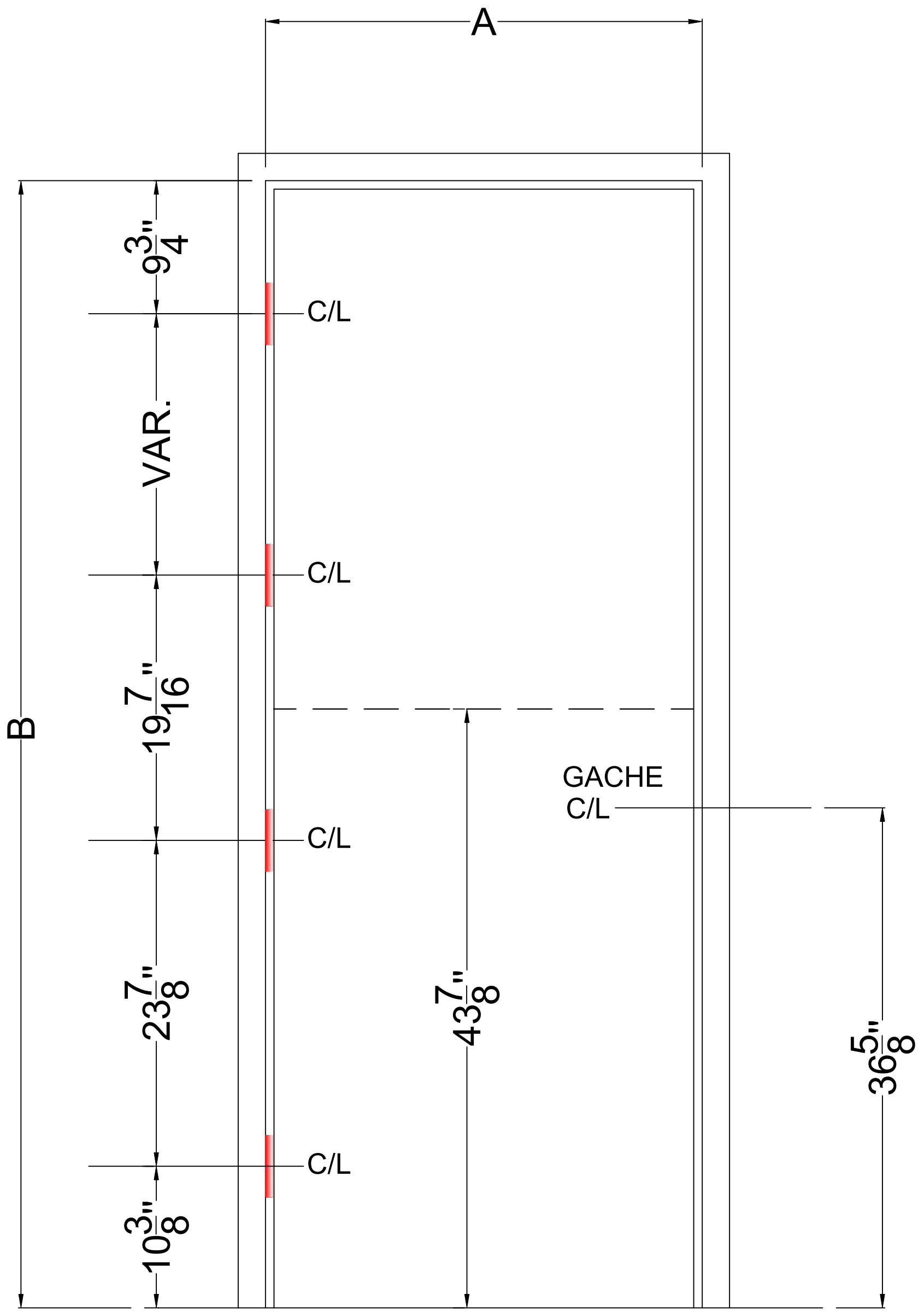
CADRE ELEVATION 1H (CADRE HOLLANDAIS)
